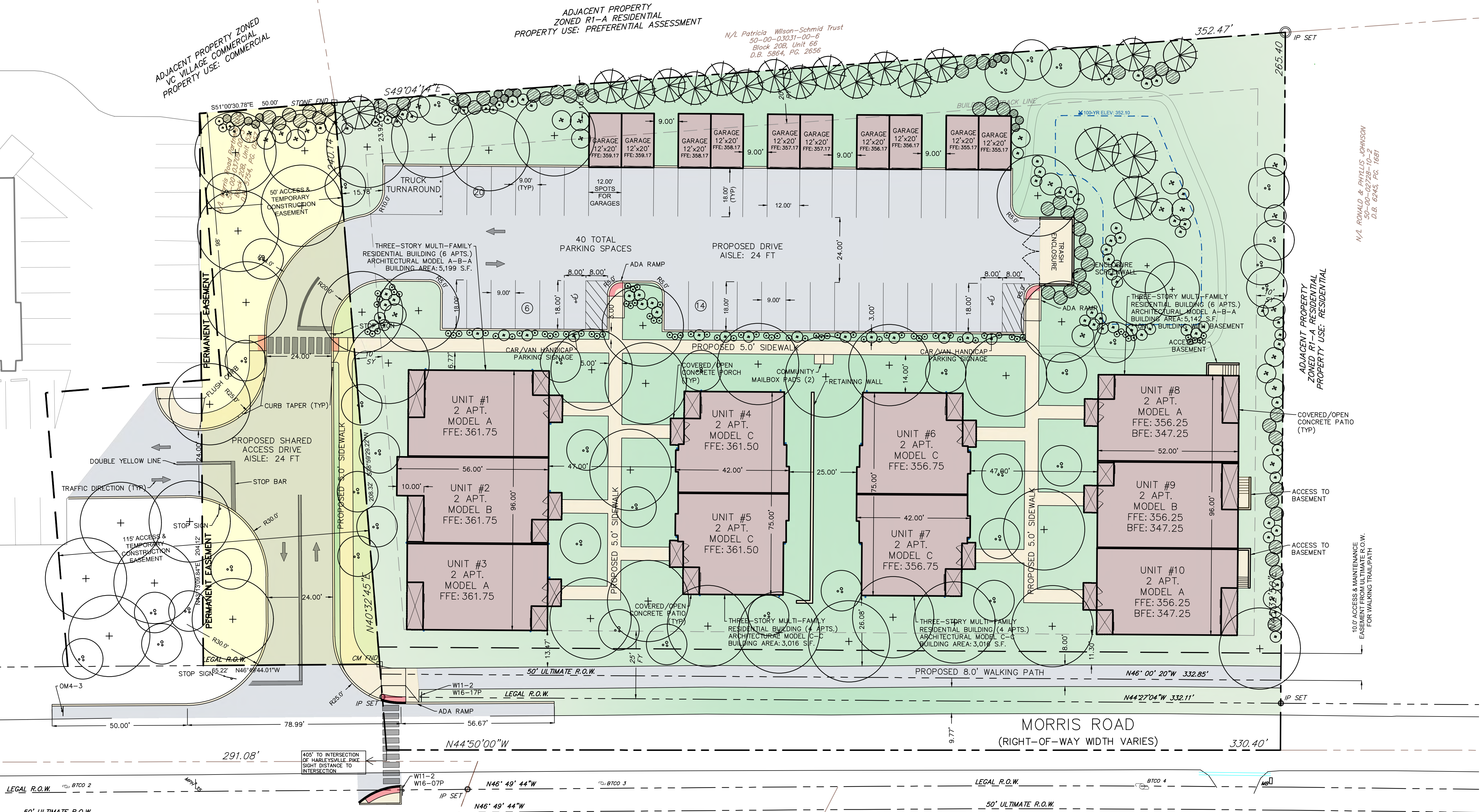
SCALE: 1" = 500'
